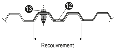
Recouvrement 2 ondes et couturage
